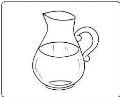
Estado líquido
