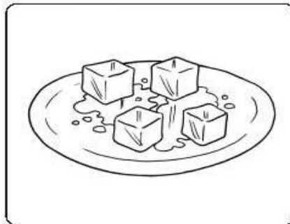
Estado sólido
